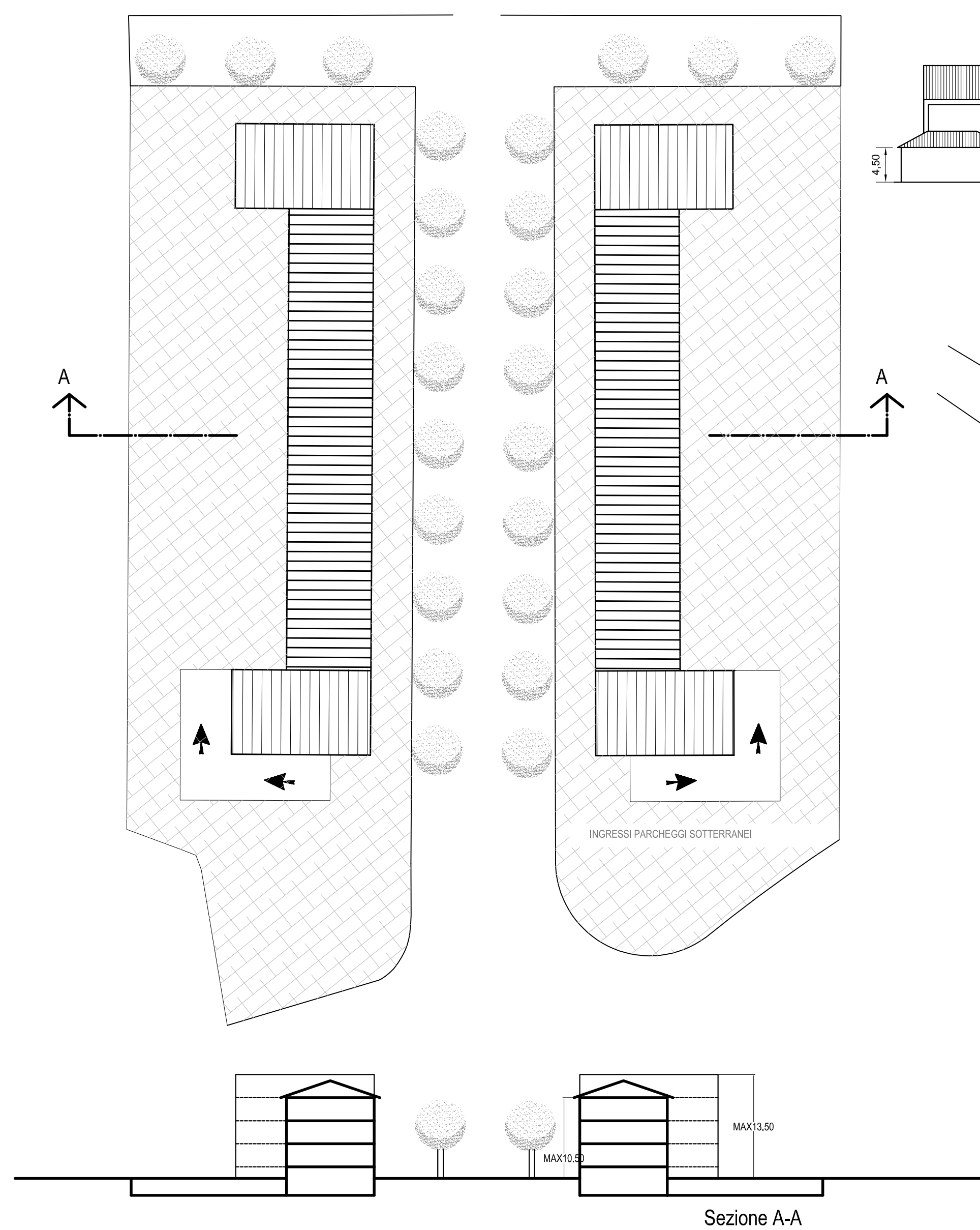
SUB AMBITO 2C SCALA 1:500
