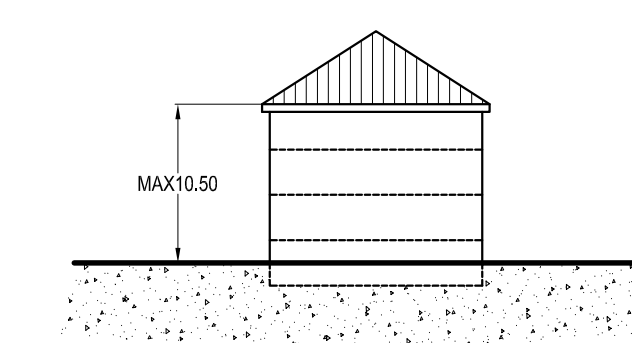
PROSPETTO A-A
